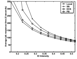
(d) Average Response Time ( \lambda = 0.008 )
